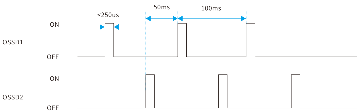
NPN输出诊断时序图：
