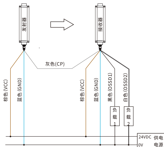
PNP接线图
