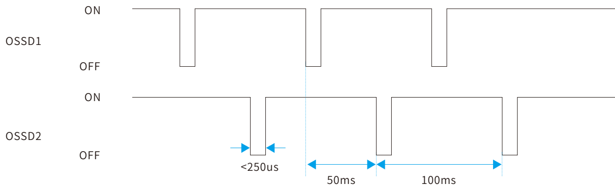
PNP输出诊断时序图：
