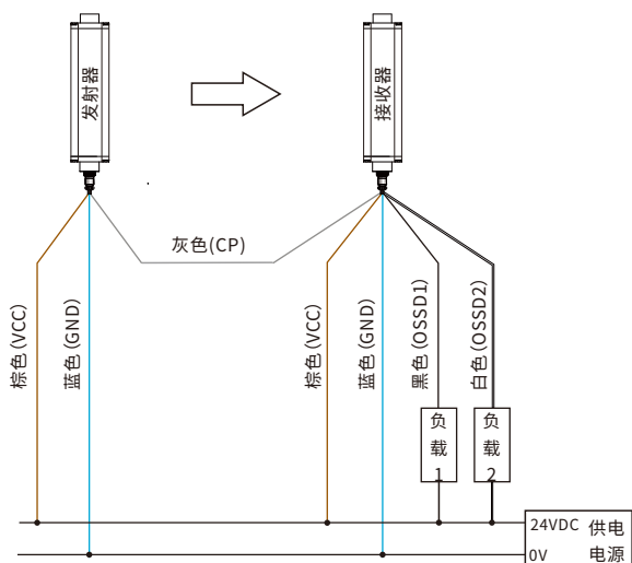
NPN接线图
