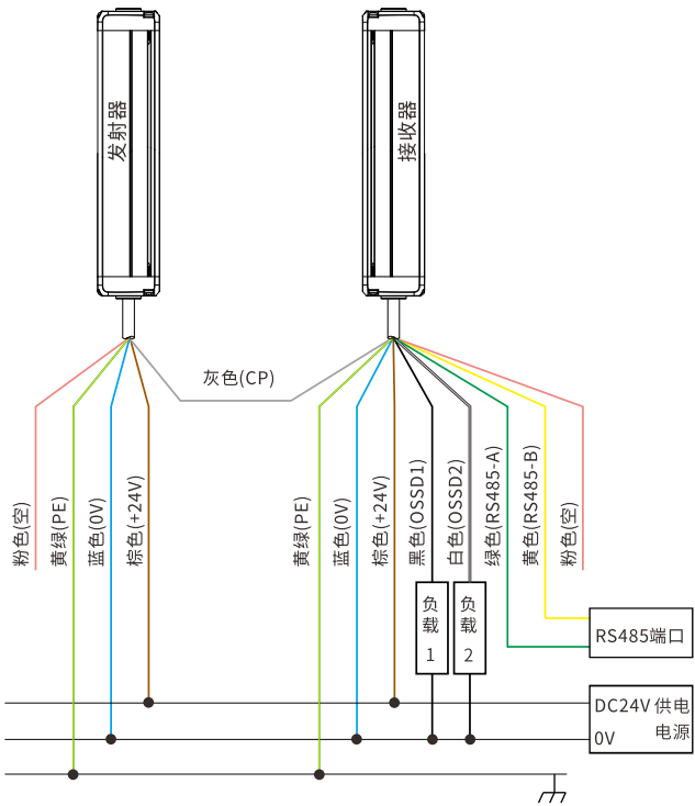
PNP接线图
