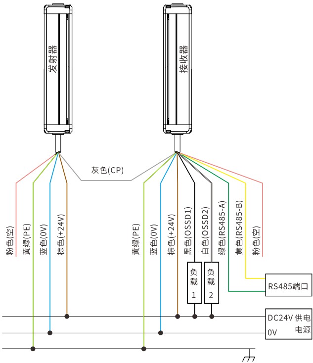
NPN接线图
