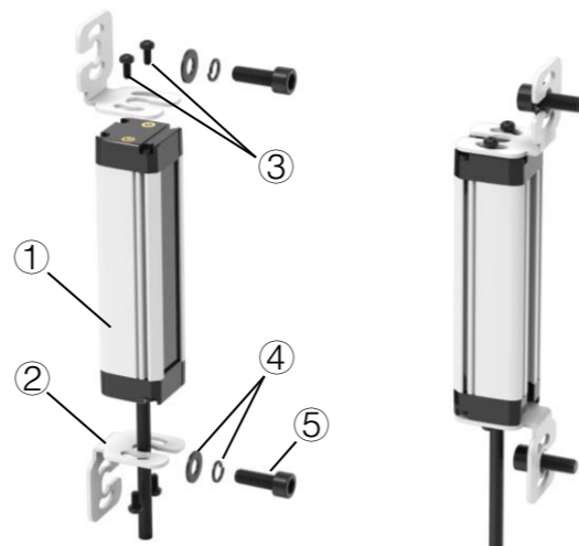
图 9-2 LD 上下支架安装示意图
