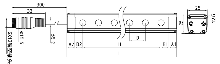
图 7-1 光栅结构尺寸示意图
