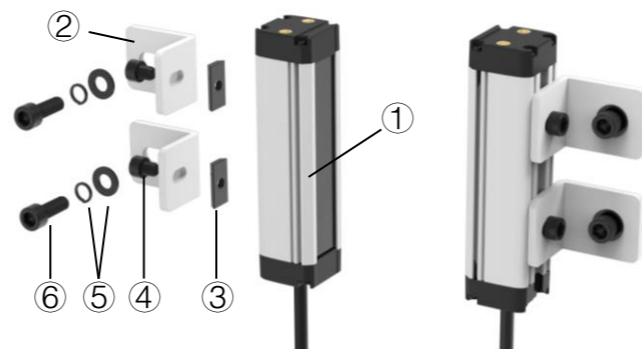
图 9-1 L 支架安装示意图
