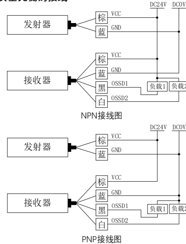
图 6-1 光栅接线示意图
