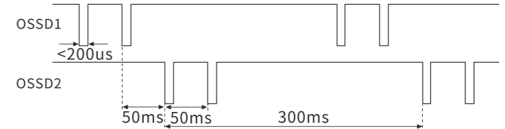
图 6-2 输出诊断时序图
