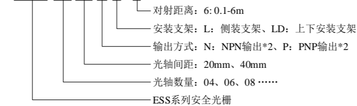
图 4-1 光栅型号说明示意图
