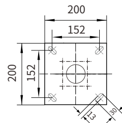
固定底板
