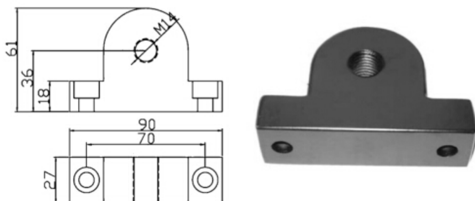
安装底座
