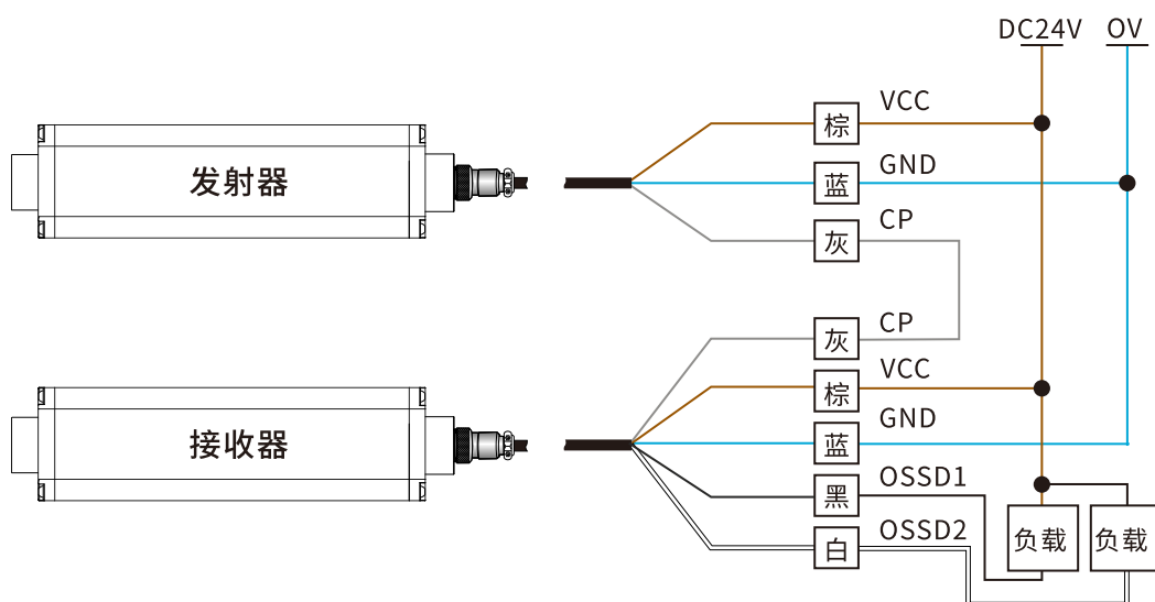
NPN接线图
