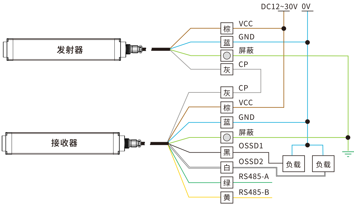
RS485输出接线图 NPN开关量输出方式
