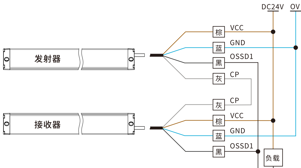
NPN接线图
